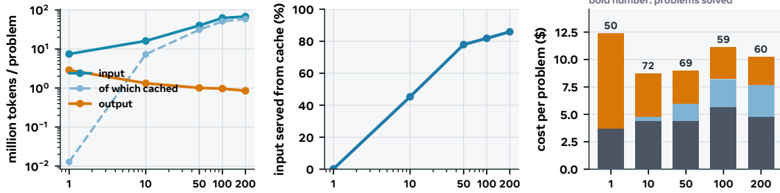
FATE-X · Gemini 3.1 Pro
