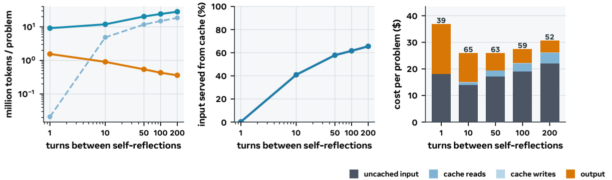
FATE-X · Gemini 3.1 Pro
